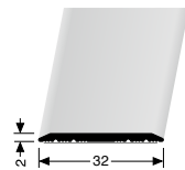
443 SK ÜBERGANGSPROFIL CONNECTING PROFILE
