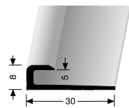
802 U ABSCHLUSSPROFIL BORDER PROFILE
