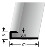
800 U ABSCHLUSSPROFIL BORDER PROFILE
