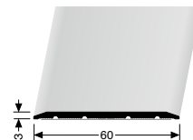
446 SK ÜBERGANGSPROFIL CONNECTING PROFILE
