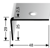
853 TREPPENKANTENPROFIL STAIR NOSING
