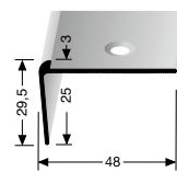
854 TREPPENKANTENPROFIL STAIR NOSING
