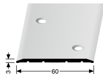
446 ÜBERGANGSPROFIL CONNECTING PROFILE
