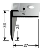
816 TREPPENKANTENPROFIL STAIR NOSING
