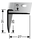
815 TREPPENKANTENPROFIL STAIR NOSING
