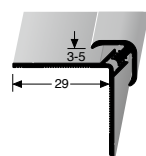
153 U 2-TEILIGE CLIP-AUSSENECKE 2-PART CLIP EXTERNAL CORNER
