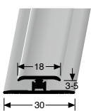
177 U 2-TEILIGER CLIP-VERBINDER 2-PART CLIP CONNECTOR
