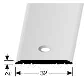
443 ÜBERGANGSPROFIL CONNECTING PROFILE
