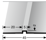
170 U VERBINDER CONNECTOR
