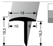
294 EINFASSPROFIL EDGE TRIM
