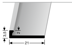
299 U ABSCHLUSSPROFIL EDGE TRIM
