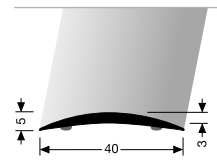
462 SK ÜBERGANGSPROFIL CONNECTING PROFILE
