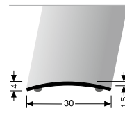
459 SK ÜBERGANGSPROFIL CONNECTING PROFILE
