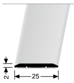
442 SK ÜBERGANGSPROFIL CONNECTING PROFILE
