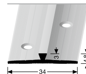
365 ABSCHLUSSPROFIL EDGE TRIM
