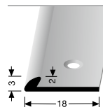
355 ABSCHLUSSPROFIL EDGE TRIM
