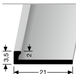
299 U ABSCHLUSSPROFIL EDGE TRIM
