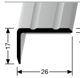
237 SK WINKELPROFIL ANGLE EDGE
