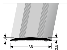
440 SK ÜBERGANGSPROFIL CONNECTING PROFILE
