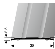
438 SK ÜBERGANGSPROFIL CONNECTING PROFILE
