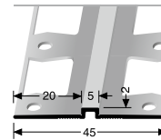
170 G VERBINDER CONNECTOR
