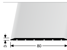
444 SK ÜBERGANGSPROFIL CONNECTING PROFILE
