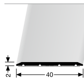
441 SK ÜBERGANGSPROFIL CONNECTING PROFILE
