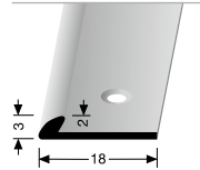
355 ABSCHLUSSPROFIL EDGE TRIM
