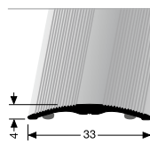
231 SK ÜBERGANGSPROFIL CONNECTING PROFILE
