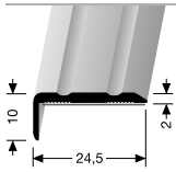
236 SK WINKELPROFIL ANGLE EDGE
